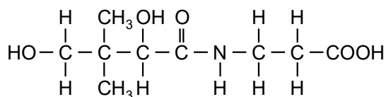
図 10 パントテン酸の構造式 (C 9 H 17 NO 5 、分子量=219.2)
